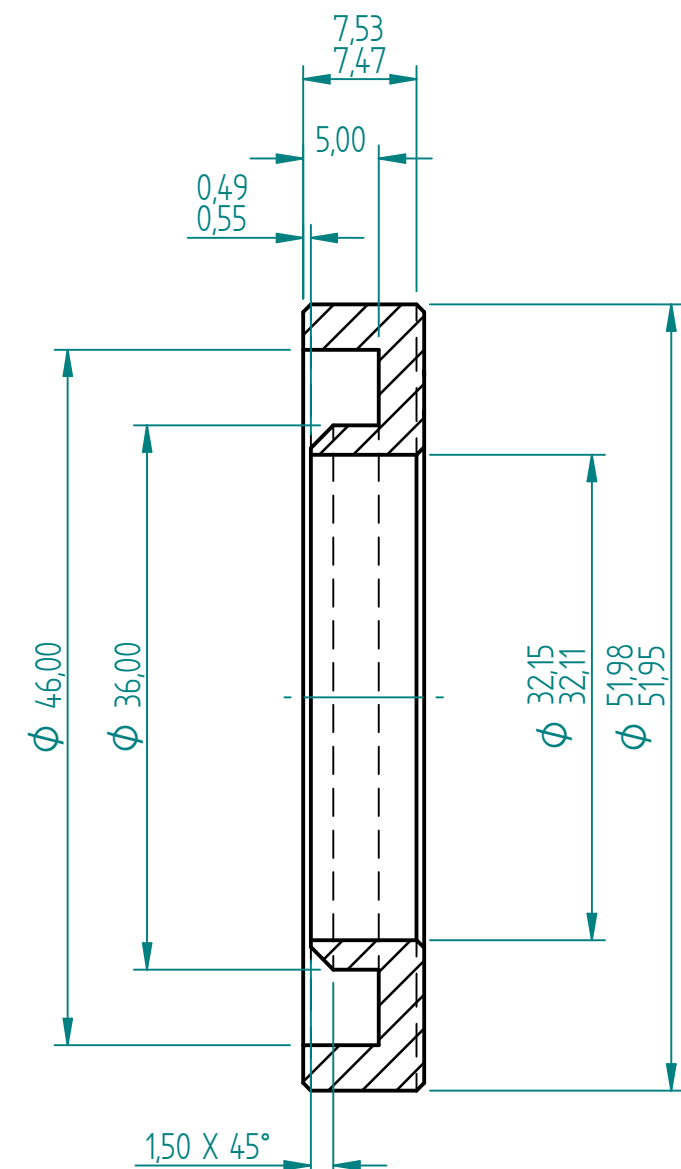
SECTION A-A
